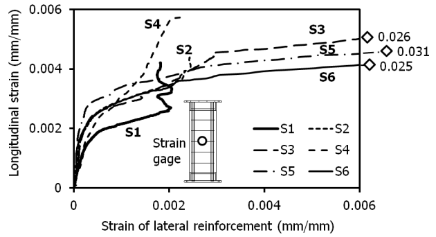
그림 10. 횡방향 철근의 변형을 계측 결과
