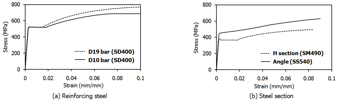
그림 3. 응력-변형률 관계
