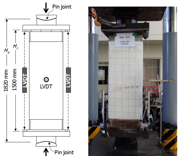
그림 5. 실험 셋팅 및 LVDT 계측
