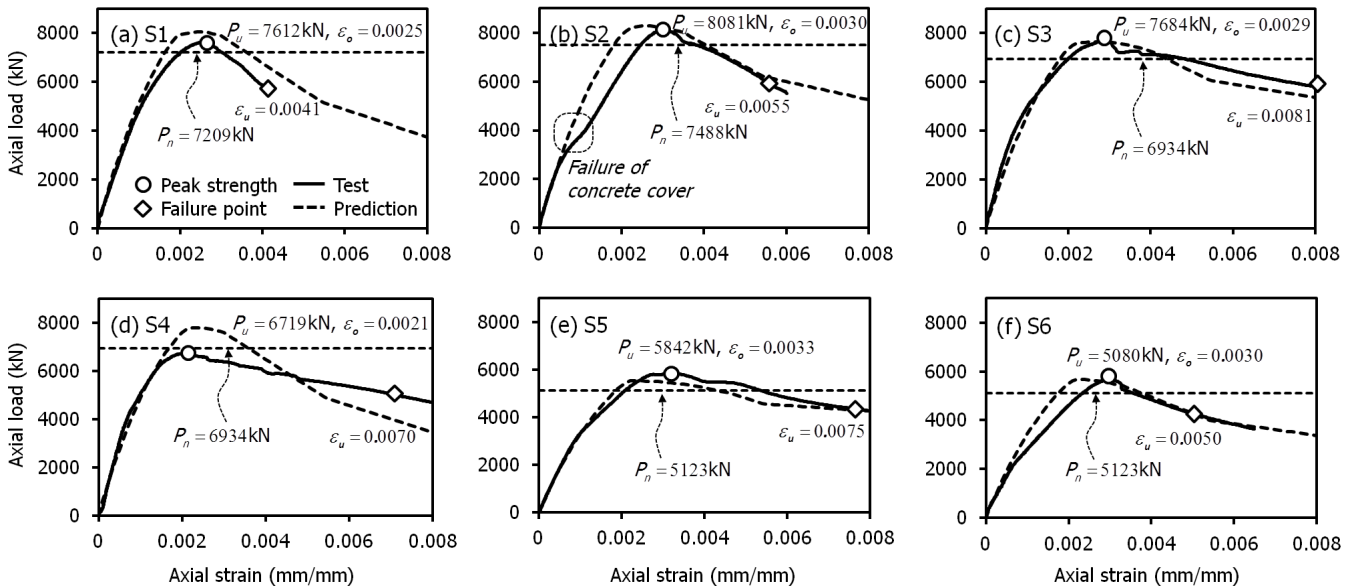
그림 6. 압축하중-변형률 관계
