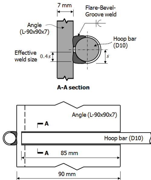
그림 4. 앵글-횡철근 용접 상세 (Flare-Bevel-Groove Weld)
