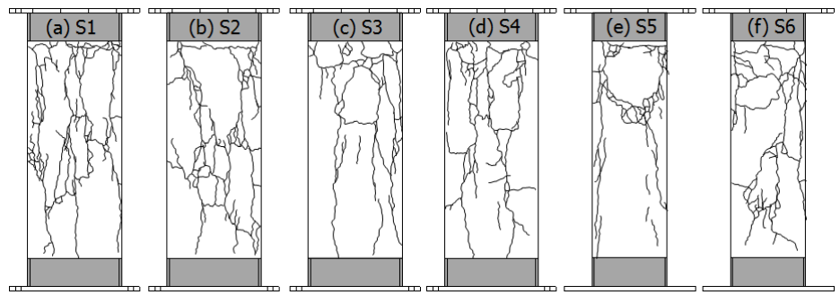
그림 8. 실험 종료 후 기둥실험체 표면의 콘크리트 균열 및 파복 파괴 양상
