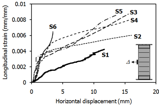
그림 9. 면외방향 수평변위
