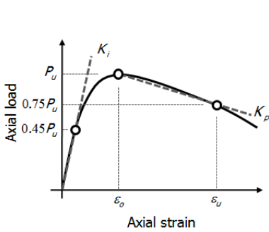
그림 7. 최대강도, 최대변형, 강성의 정의
